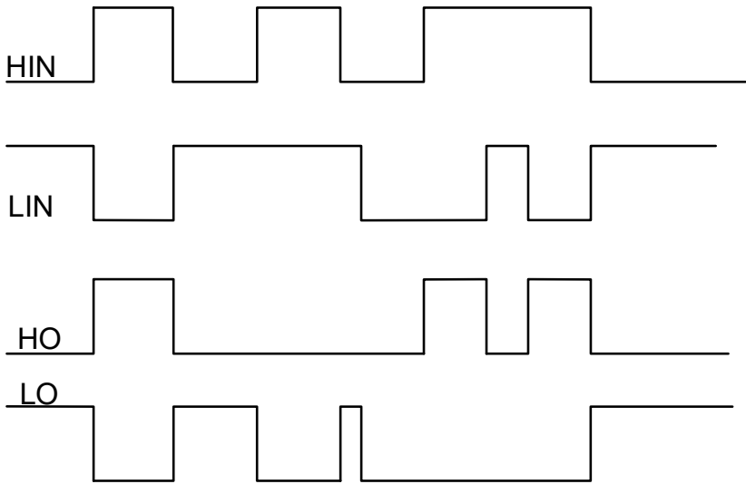
图 9-1 HM2101K 输入输出时序波形
